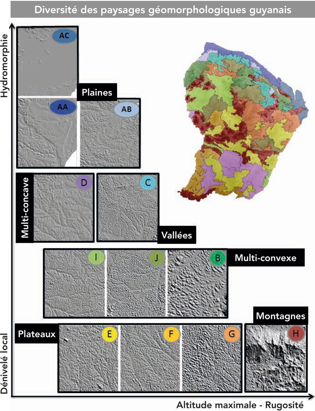
Figure 6 : Diversité des reliefs illustrée par des extraits du SRTM 30 m (image radar de 20 km x 20 km - les couleurs de la carte correspondent à celles des pastilles). Sur les plateaux, le réseau hydrographique très enfoncé, orienté et hiérarchisé quadrille des reliefs larges et anguleux donnant un aspect de papier froissé. Le réseau est moins enfoncé sur les reliefs multi-concaves qui sont aussi plus hydromorphes. Les reliefs sont plus arrondis
