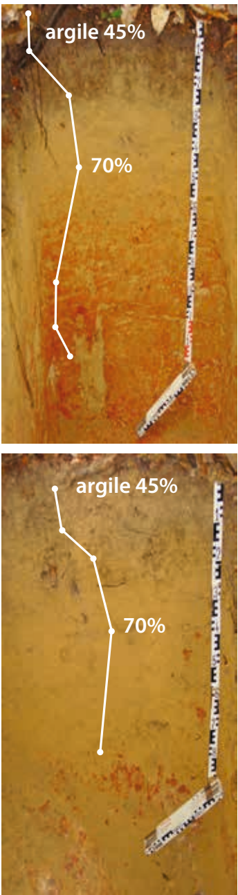
Fosses ouvertes sur le site de Crique Plomb par D. Paget (2000) et profils décrits par V. Freycon, D. Paget et M. Jamagne - en haut, acrisol ferrique - en dessous, acrisol plinthique sur cuirasse démantelée (les blocs de cuirasse forment des taches rouges) - en surimpression la courbe d'évolution du taux d'argile sur les profils (courbes en forme de « ventre »).
