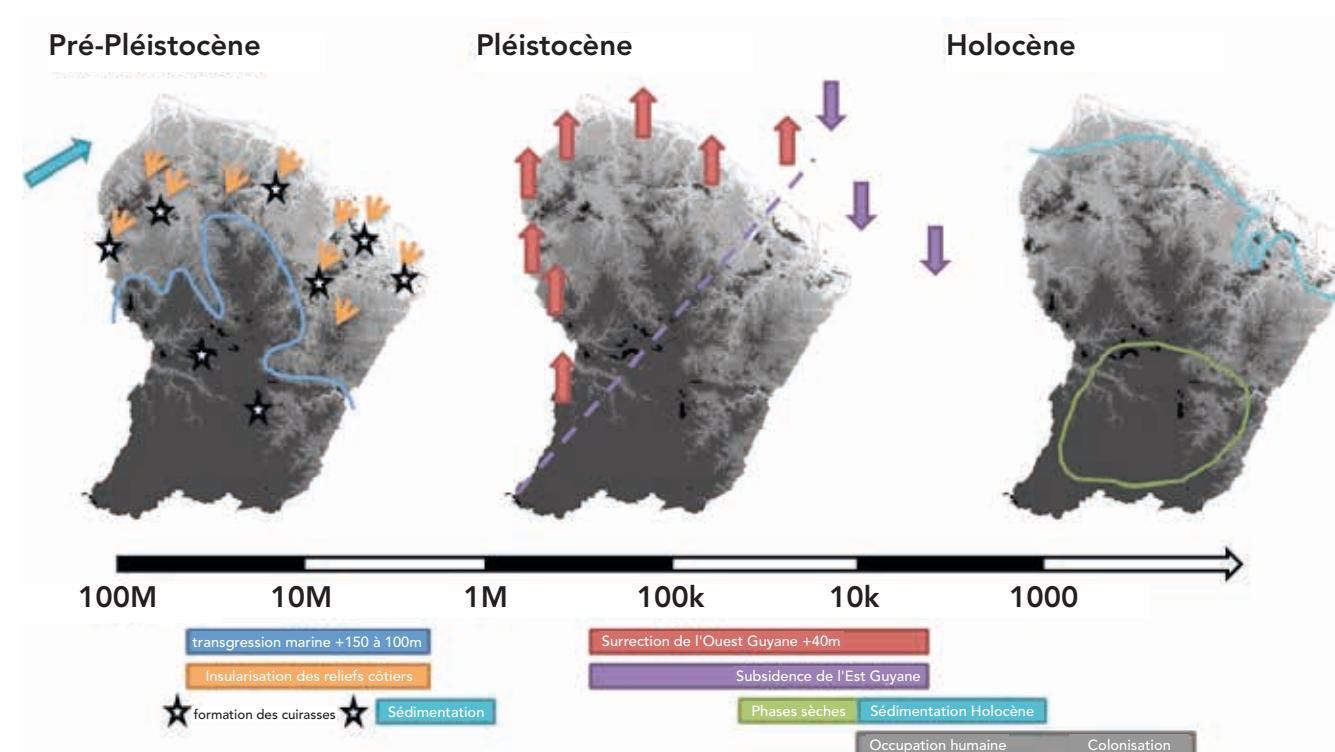
Figure 5 : Chronologie schématique des événements géologiques, climatiques et marins ayant façonné les paysages et formations végétales de Guyane – Les codes couleurs utilisés sur les cartes correspondent aux événements indiqués sur la frise (adapté de Nores 1999 [31], Palvadeau 1998 [37], Duputie et al. 2009 [60]).
