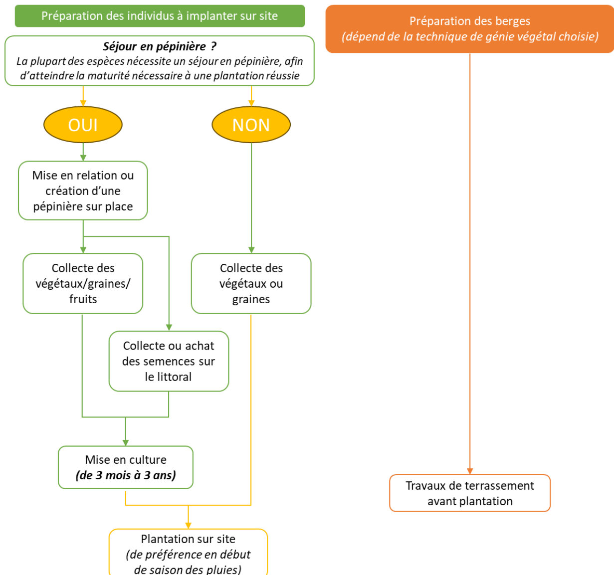
Figure 7 : Principes généraux de mise en œuvre de technique de génie végétal
