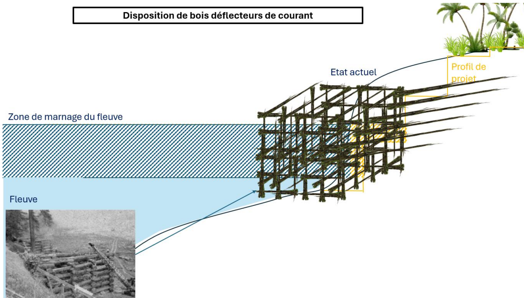
Figure 16 : Schémas de principe d'utilisation de bois mort pour le confortement de berge en Guyane
