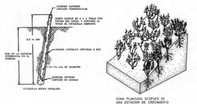
Figura 4.2. Detalle del uso de la técnica de estacado Fuente: López y Mataix, 1999
