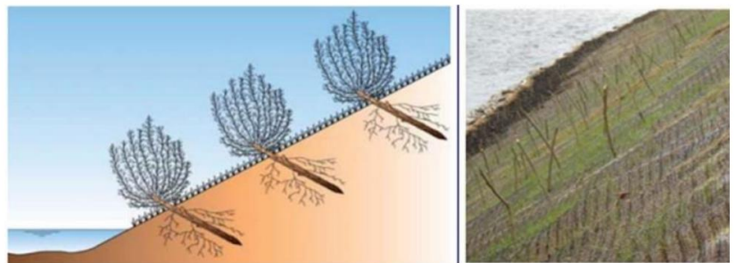
Figura 22..Esquema de estacado (izquierda) y estacado en el río Nalón a su paso por Asturias (derecha). Fuente: (Ministerio de Medio Ambiente y Medio Rural y Marino, 2011).
