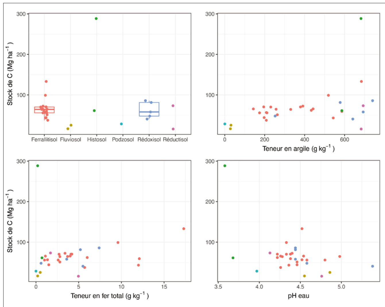
Figure 12 : Stocks de C du sol (0-30 cm) sur les sites RMQS de Guyane selon le type de sol, la teneur en argile, la teneur en fer total, et le pH mesuré dans l'eau.
